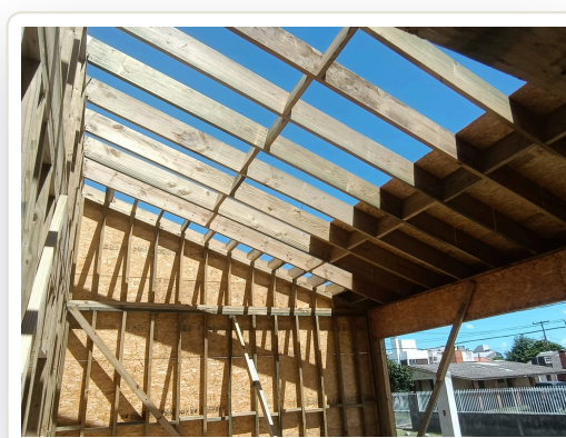
Estrutura em Wood Frame durante execução — o mesmo rigor técnico aplicado na manutenção
